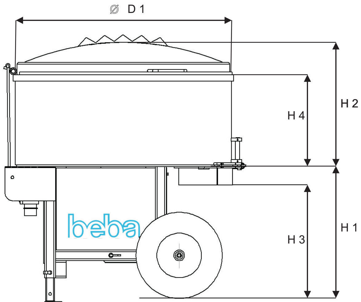
B 1200 Maßblatt
