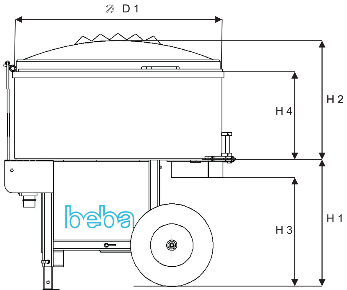
B 1500 Maßblatt
