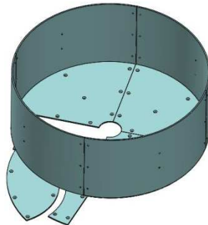
Verkleidung-Hardox
