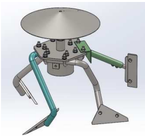
B325-Standardmischwerkzeug
